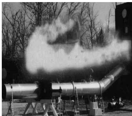
Obr. 6: Vypouštění přetlaku z výbuchu
