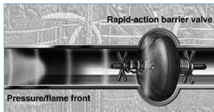
Obr. 8: Protivýbušná izolace s rychle reagujícím tlumičem
