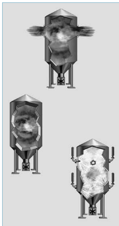
Obr. 5: Zadržení výbuchu (vlevo), odlehčení výbuchu (nahore) a potlačení výbuchu (dole vpravo) pomocí vhodné konstrukce zařízení
